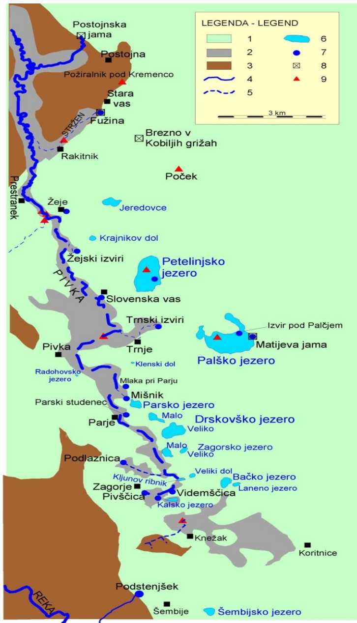
Slika 2: Hidrogeološka karta območja reke Pivke in presihajočih Pivških jezer.
