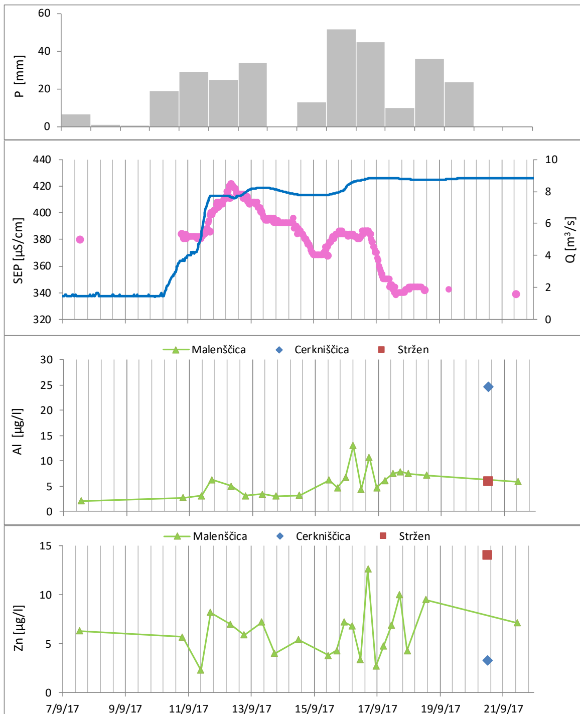
Slika 12: Analiza sprememb vsebnosti izbranih kovin (aluminij – Al in cink – Zn) v izviro Malenščica v času vodnega vala v septembru 2017. Prikazane so dnevne padavine na ARSO postaji Postojna (P), pretoki izvira Malenščica (Q) in vrednosti specifične električne prevodnosti (SEP) v izviro Malenščica. Analiza vsebnosti Al in Zn izven vplivnega območja vadišča je bila opravljena v Cerknjščici in Strženu 20.9.2017.
